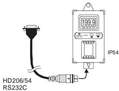
HD206-1 Sensori di temperatura ed umidità relativa esterni
