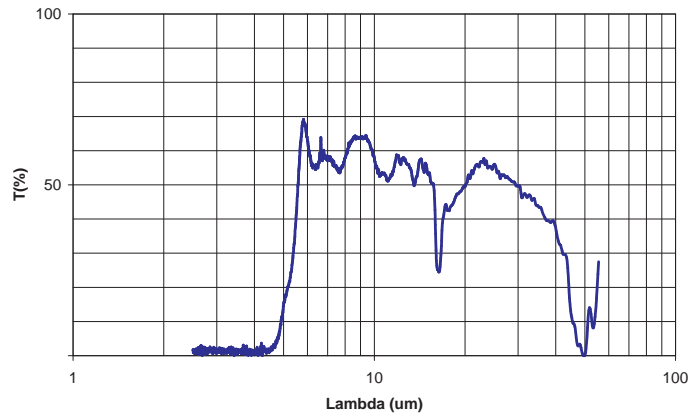
Grafico 1: Trasmissione della finestra in silicio.
