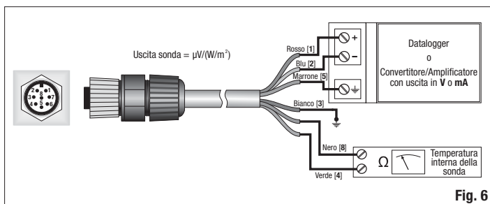
Figura 6: esempio di collegamento del pirgeometro
