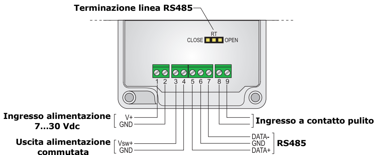
Fig. 3.7.1: connessioni LR35[L]W-MB
