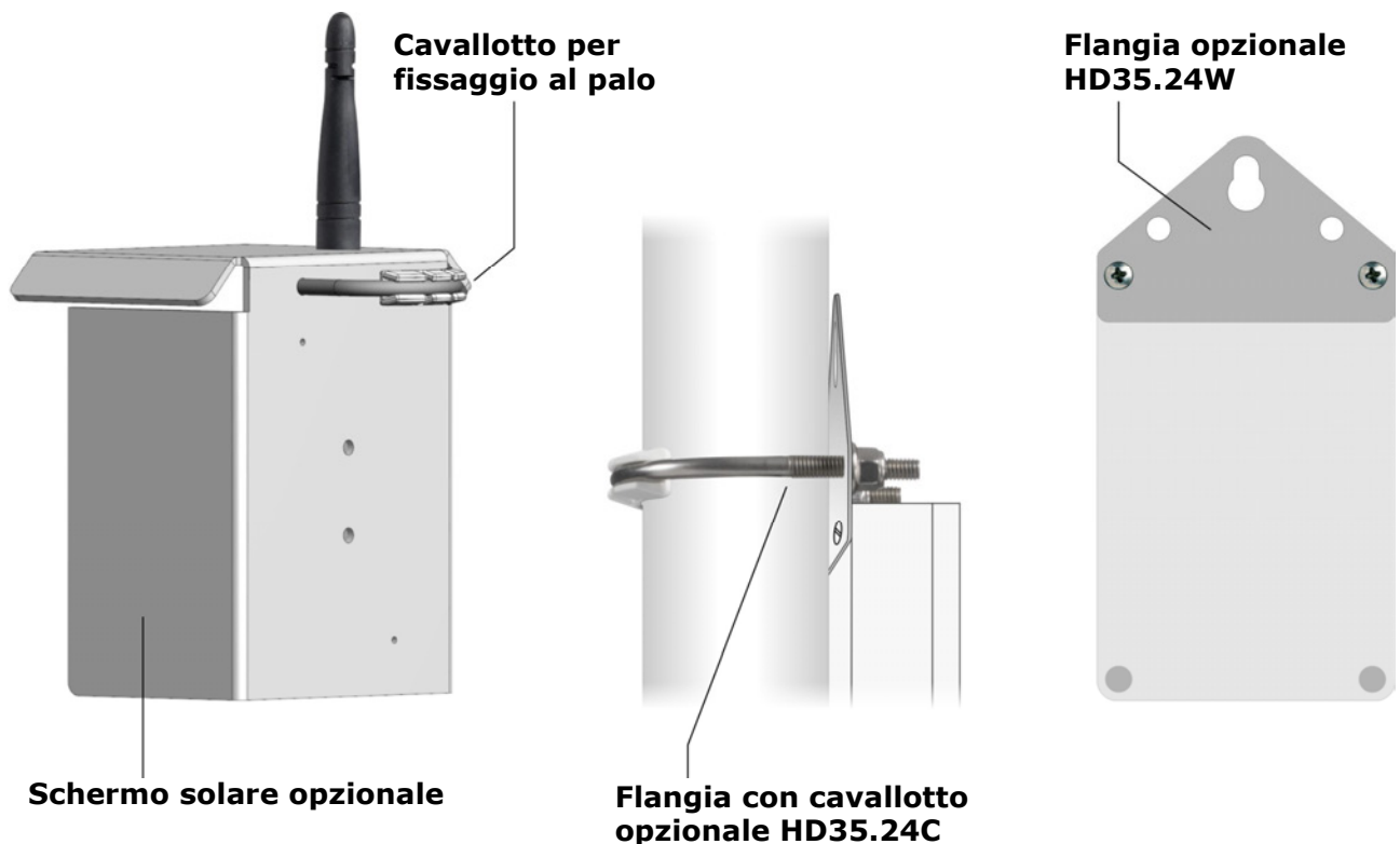
Fig. 3.3.2: modalità di installazione modelli per esterni
